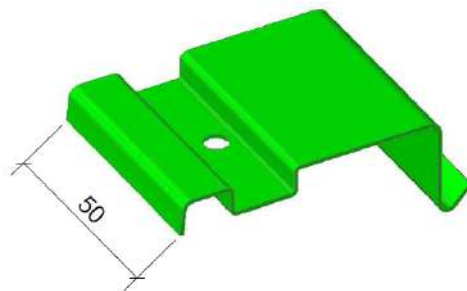
DETALLE 3D GRAPA FIJACIÓN HIANSA
