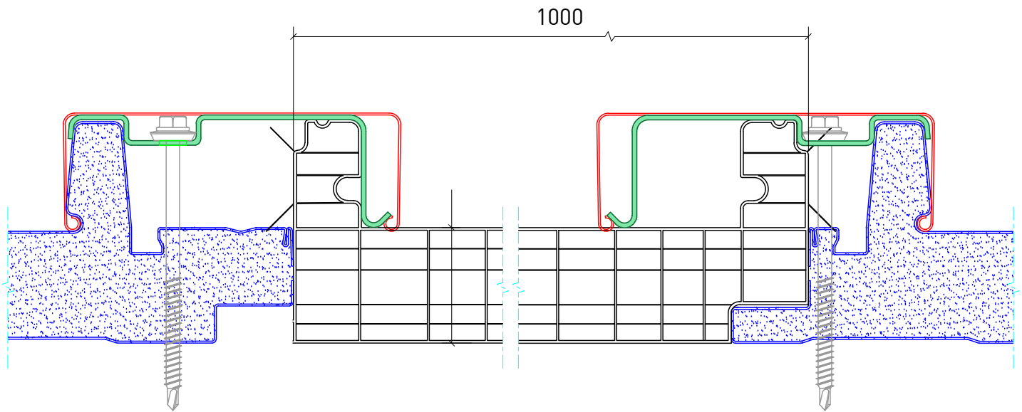
DETALLE ENTREGA POLICARBONATO - PANEL DE CUBIERTA HIANSA 2GR/3GR
